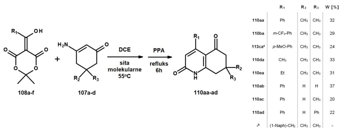
Rys.56. Seria synteza „one-pot” w kierunku otrzymania pochodnych 7,7-dimetylo-4-fenyl-7,8-dihydrochinolin-2,5(1H,6H)-dionu ( 110aa-ad ); a produkt o innej konstytucji; b rozpad enamidu po dodaniu PPA
