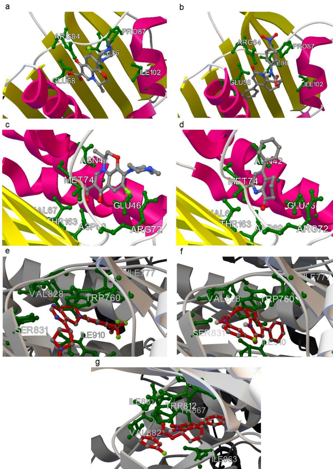
Rys.33. Wyniki dokowania molekularnego dla pochodnych 4-fenyl-5,6,7,8-tetrahydrochinolin-2(1H)-onu: (a) wiązanie lewofloksacyny do gyrazy Staphylococcus aureus (PDB: 3G75) 167 ; (b) wiązanie 94b do gyrazy Staphylococcus aureus (PDB: 3G75); (c) wiązanie lewofloksacyny do topoizomerazy IV Escherichia coli K-12 (PDB: 3FV5) 168 ; (d) wiązanie 95 do topoizomerazy IV Escherichia coli K-12 (PDB: 3FV5); (e) wiązanie Leniolisibu do PI3K \delta (PDB: 5O83) 169 ; (f) wiązanie 94d do PI3K \delta (PDB: 5O83); (g) wiązanie 94d do PI3K \gamma (PDB: 3OAW) 170
