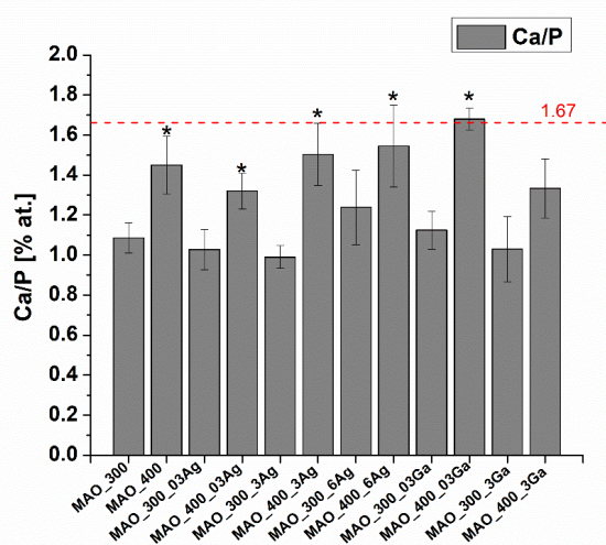
Rysunek 26 Stosunek wapnia do fosforu dla różnych parametrów wytwarzania warstw MAO wraz z zaznaczeniem wartości stechiometrycznego hydroksyapatytu ( n = 3 ; dane to średnie \pm SD ; * istotnie różne między grupami napięcia, p < 0.05 )
