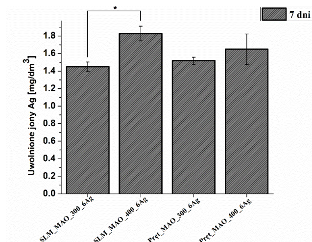
Rysunek 45 Uwolnienie jonów srebra do PBS po 7 dniach inkubacji z warstw MAO wytworzonych przy różnych parametrach procesu na materiale macierzystym wytworzonym metodą SLM oraz na materiale macierzystym w postaci komercyjnego pręta walcowanego na gorąco ( n = 6 ; dane to średnie \pm SD; * istotnie różne między grupami napięcia, ( p < 0,05 ))
