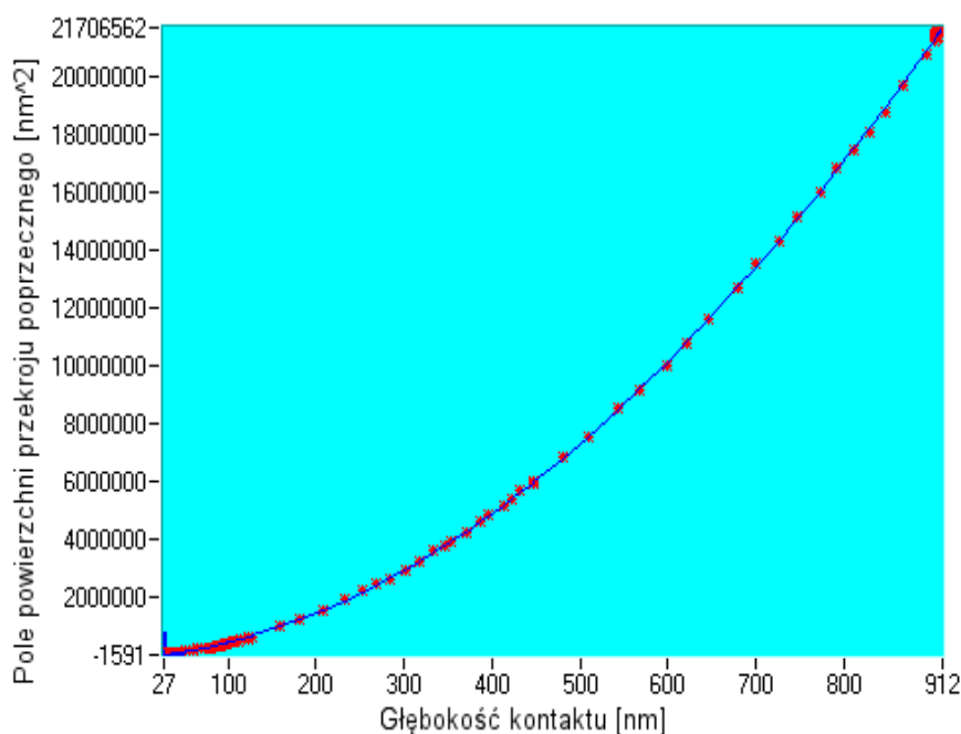
rys. 6.3. Zbiór pomiarów funkcji kształtu wgłębnika (kolor czerwony) oraz krzywa wielomianowa 3-go stopnia dopasowana do punktów (kolor granatowy). Pomiarzy wykonano w próbce referencyjnej z krzemionki topionej. Opracowanie własne.
