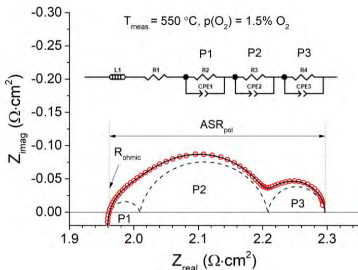
Rysunek 15. Wyniki widma impedancyjnego wraz z dopasowaniem układu zastępczego przedstawione w formie wykresu Nyquista dla elektrody LSCF modyfikowanej 400 nm warstwą LSC pomiędzy elektrolitem i elektrodą zmierzoną w temperaturze 550°C i ciśnieniu parcjalnemu tlenu 1.5% O 2 [117].
