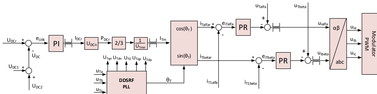
Rys.4. Schemat blokowy układu sterowania przekształtnikiem T: $f_{pwm} = 20$ kHz; $f_{sam} = 20$ kHz; regulatory (nastawy), PI($U_{DC}$): $K_p = 2,7$; $T_i = 0,007$; PR($i_{T\alpha}$, $i_{T\beta}$): $K_p = 1,75$; $K_{ri} = 110$; $K_{si} = 0,005$
