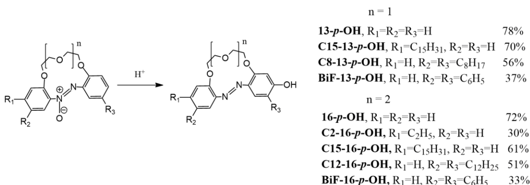
Rys. 2.26. Przegrupowanie analogiczne do przegrupowania Wallacha dla makrocyklicznych, podstawionych w pierścieniach benzenowych, azoksyzwiązków wraz z wydajnościami [27,55]
