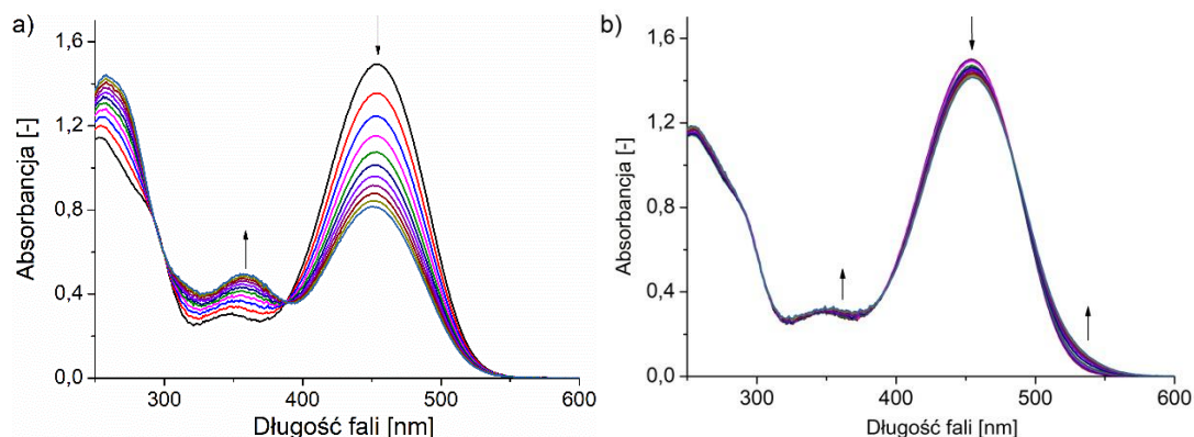
Rys. 4.40. Zmiany w widmie absorpcyjnym związku BiF-19-p-OH ( 4,34 \cdot 10^{-5} \text{ mol/dm}^3 ) podczas miareczkowania roztworem chloranu(VII) a) sodu ( c = 0-6,11 \cdot 10^{-4} \text{ mol/dm}^3 ), b) magnezu ( c = 0-2,40 \cdot 10^{-3} \text{ mol/dm}^3 ) w acetonitrylu
