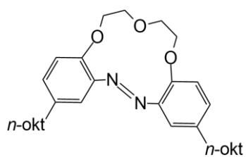
n-okt-13-Azo
