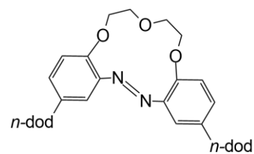
n-dod-13-Azo
