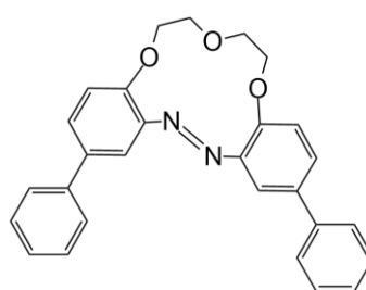
BiF-13-Azo
