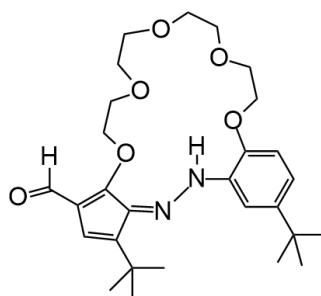
t-Bu-19-al
