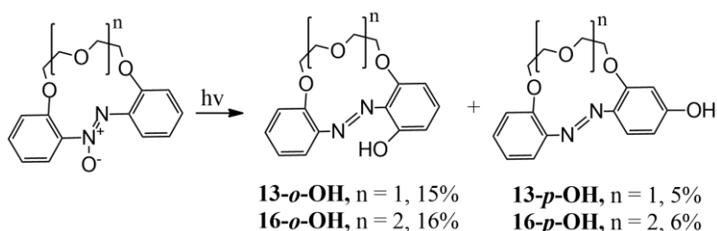
Rys. 2.27. Przegrupowanie fotochemiczne 13- oraz 16-członowej azoksybenzokorony [27]
