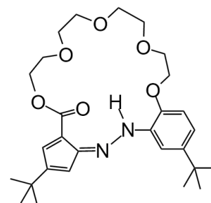
t-Bu-20-ester
