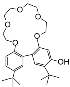
t-Bu-17-p-OH
