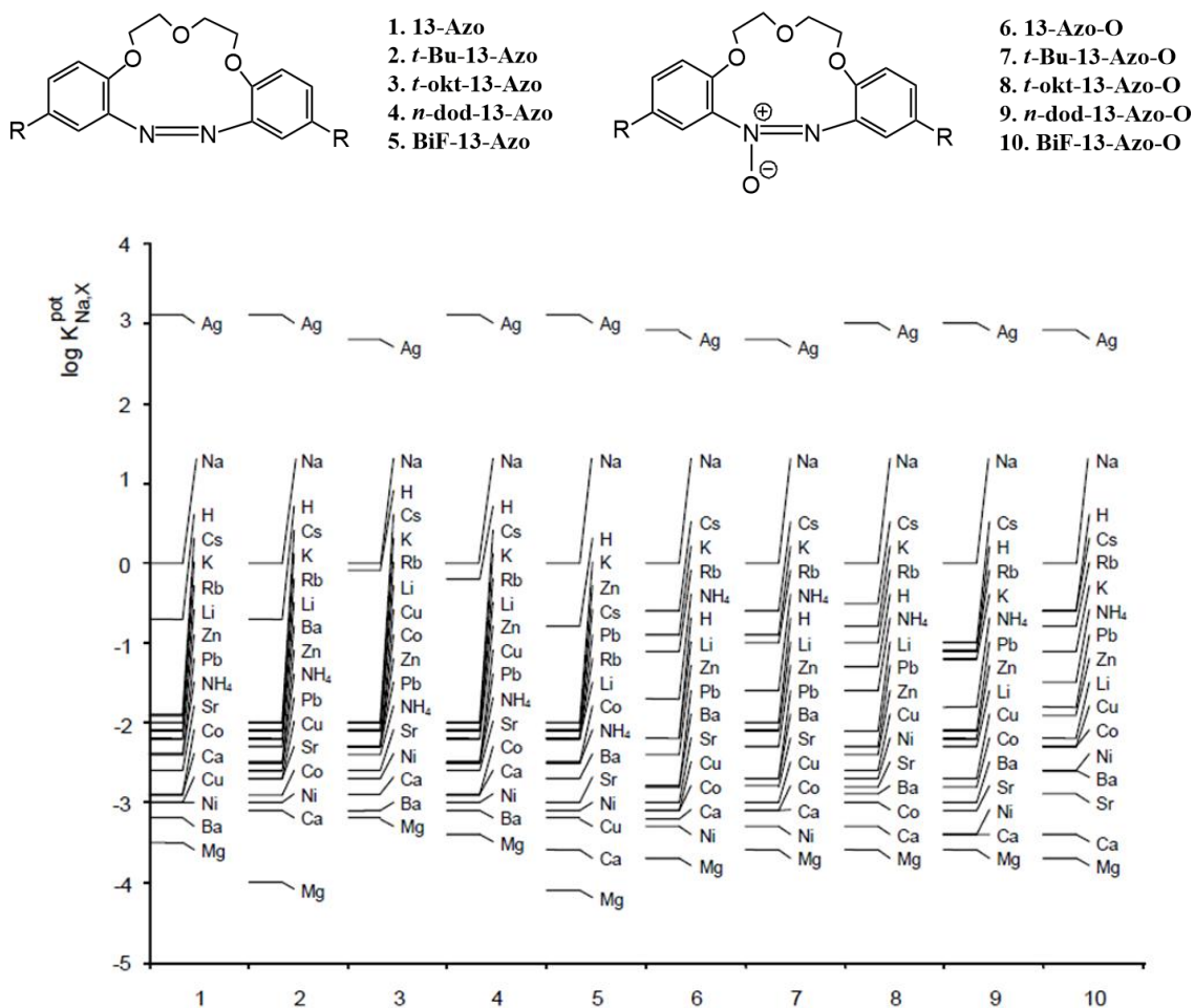
Rys. 2.17. Wartości potencjometrycznych współczynników selektywności elektrod zawierających 13-członowe azobenzokorony i azoksybenzokorony jako jonofory [14,25,33]
