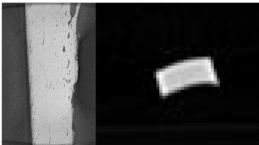
Rys. 6.14 Przykładowe obrazy, wyniki skanowania tej samej próbki kostnej. Po lewej obraz z mikrotomografu w obszarze pomiarowym, po prawej wynik skanowania tomografem klinicznym (opracowanie własne).
