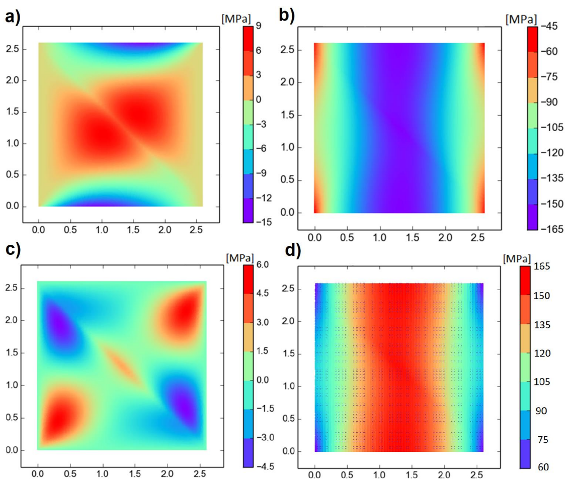
Rys. 5.24 „Wynik dokładny” obliczeń wytrzymałościowych całej próbki poddanej obciążeniu wzdłuż osi pionowej próbki. a) naprężenia normalne X b) Y c) naprężenia styczne XY d) naprężenia wg. Von Misesa. Siatka podziału 61 x 61, element 8-mio węzłowy, model własny (opracowanie własne).
