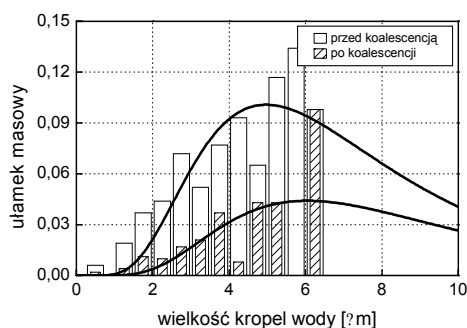
Rys. 9. Rozkład wielkości kropeł wody w oleju, złożo 40\text{--}100 \mu\text{m} , wysokość 0,12 \text{ m} , temperatura 60 \text{ }^\circ\text{C}
