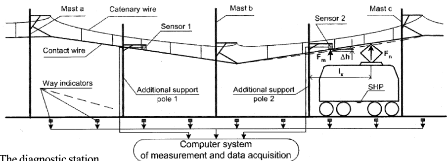
Fig. 5. Idea of the vertical force measurement on checking section Rys. 5. Koncepcja sieciowego przęsła pomiarowego
