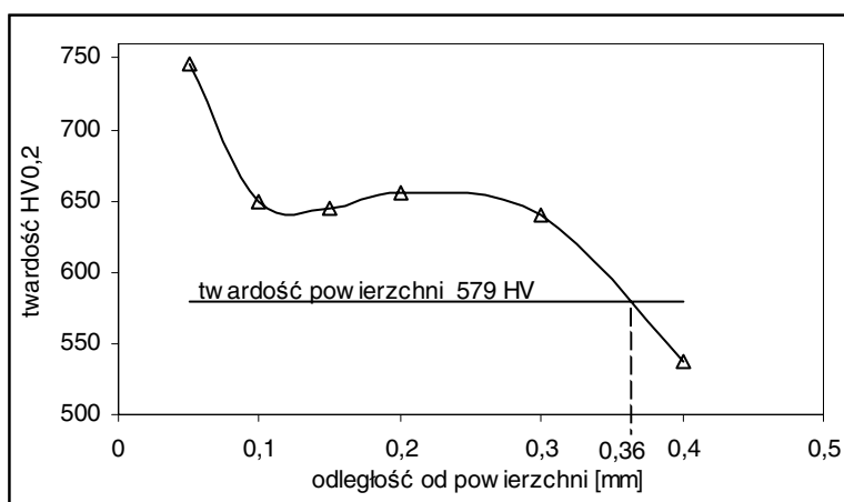
Rys. 8. Profil mikrotwardości warstwy wierzchniej napiny Fe-Cr-Mn po 70 min działania obciążeń kawitacyjnych
