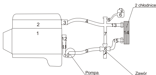
Rys. 8. Przykładowy podział obiegu chłodzenia na niezależne magazyny energii Fig. 8 Engine cooling system division for independent energy storage elements
